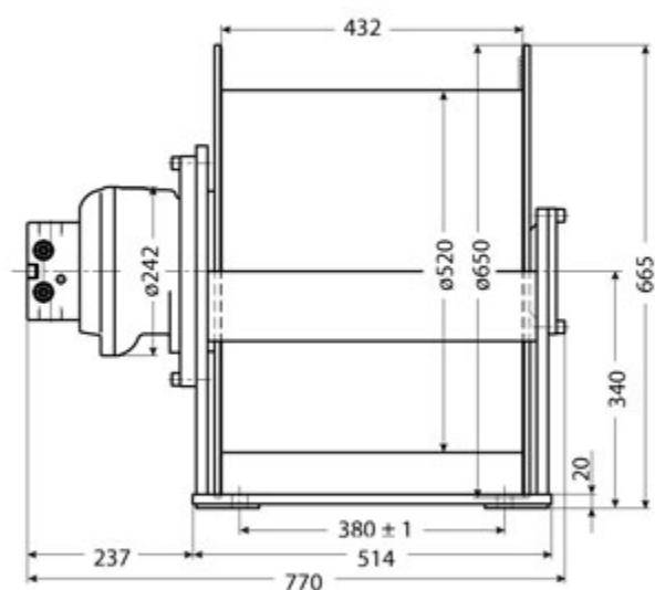
Dimensions in mm / Dimensiones en mm
